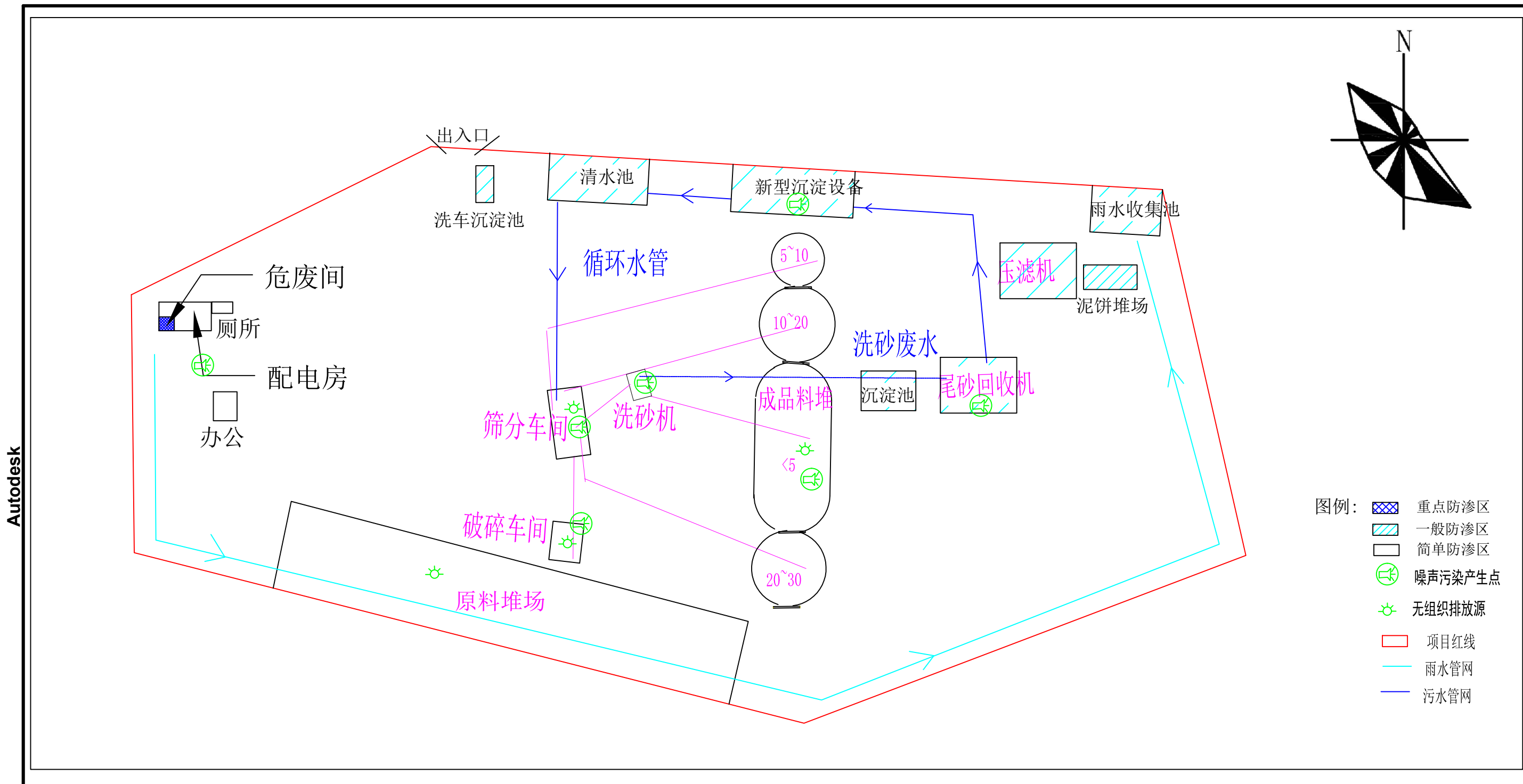
附图5 本项目总平面布置、产污节点及分区防渗图
